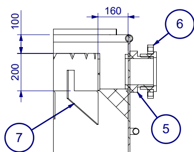
SEZIONE A-A SCALA 1 : 20
